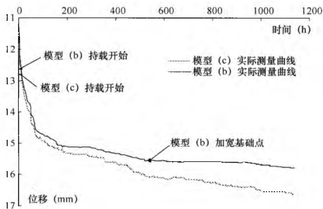
图 3 基础板(b)和(c)在持载时位移随时间发展情况
