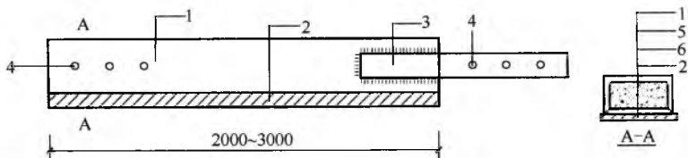
图 6 组合式下轨道板
