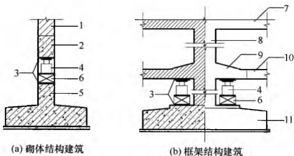
图 7.3.3-2 顶升梁、千斤顶、底座布置
