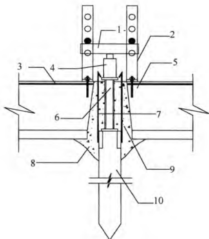
图8 预加反力封桩示意
