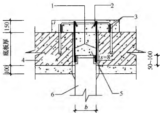
图 7 锚杆静压桩封桩节点示意
